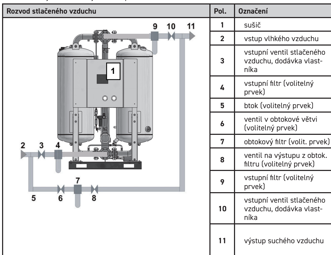
Příklad montáže s obtokovou větví
