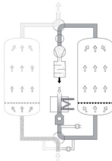
Fáze ohřevu
