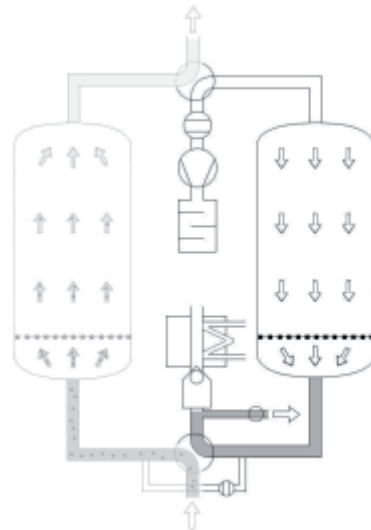
Fáze odtlakování/expanze
